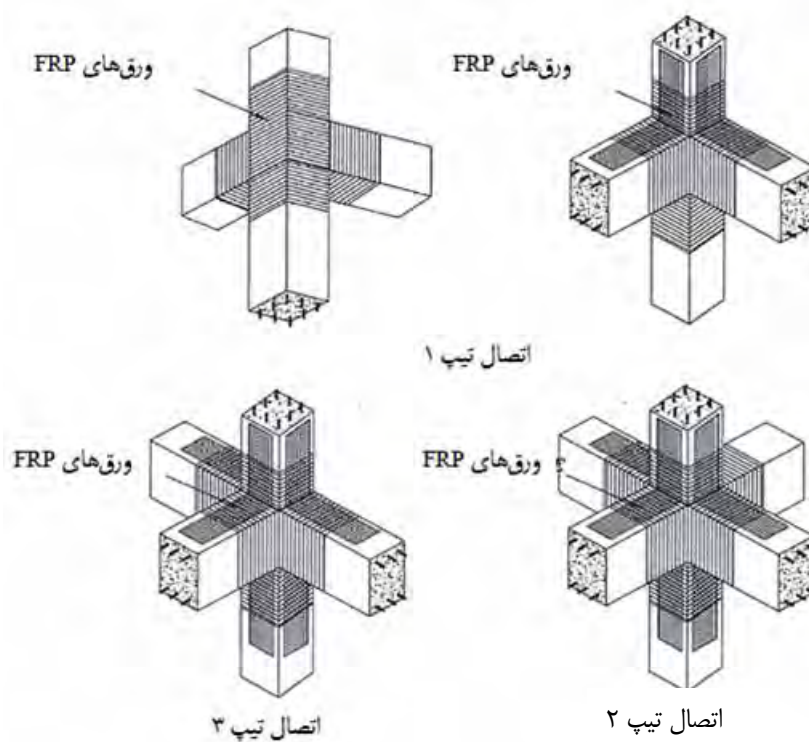
شکل ۲-۶-۳ جزئیات تپ استفاده از FRP در مقاوم‌سازی اتصالات
