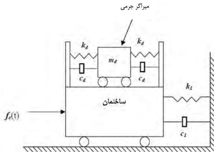
شکل ۷-۲۱- مدل میراگر جرمی در ساختمان
