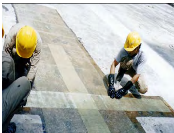
شکل ۱۱-۳-۲- مقاوم‌سازی دال در لنگرهای منفی بوسیله FRP
