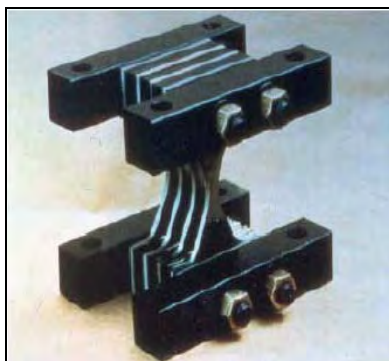
شکل ۷-۹- میراگر X-ADAS
