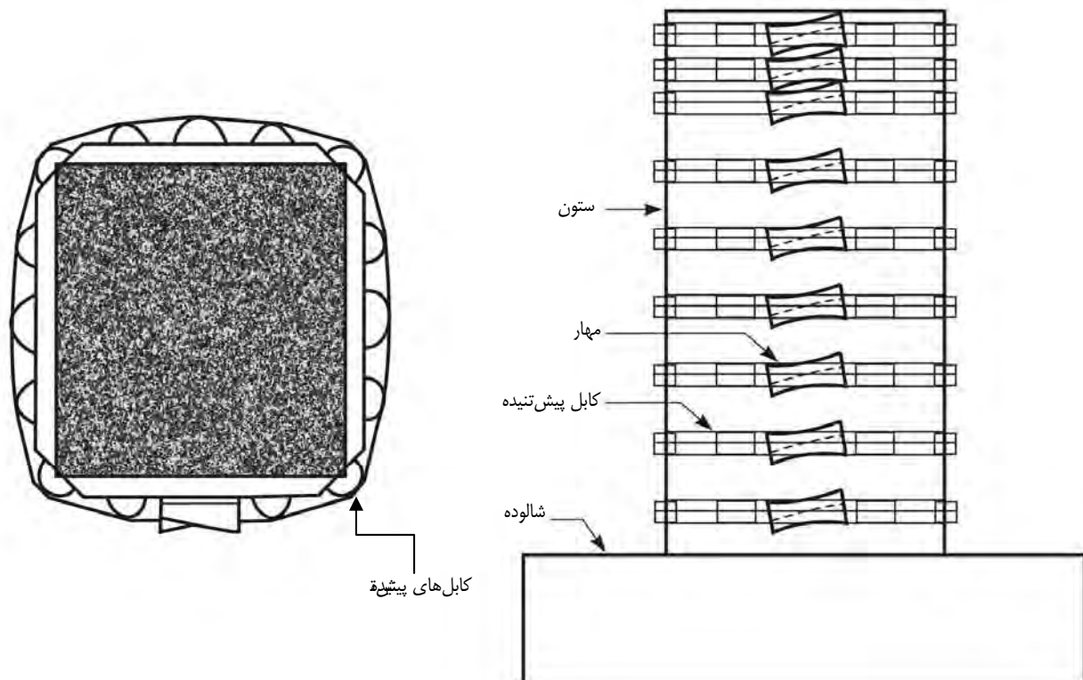
شکل ۲-۵-۱۵- استفاده از پیش‌تندگی عرضی در بهسازی ستون‌ها
