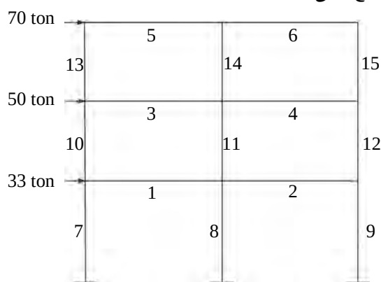
شکل ۳-۴ - توزیع نیروی زلزله در ارتفاع
