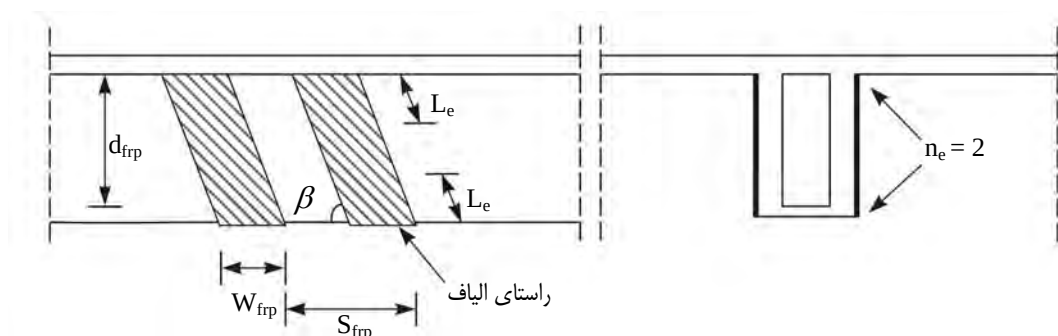
الف- تقویتی‌های برشی FRP بر وجوه جانبی
