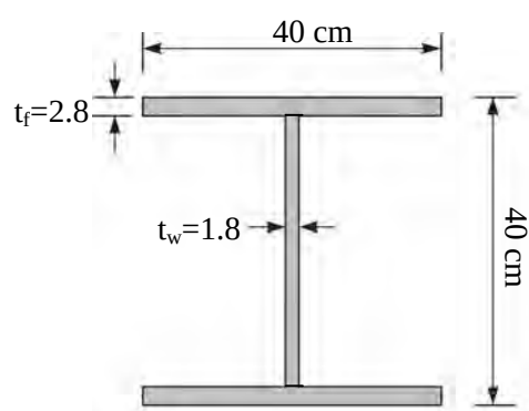
مقطع ستون
