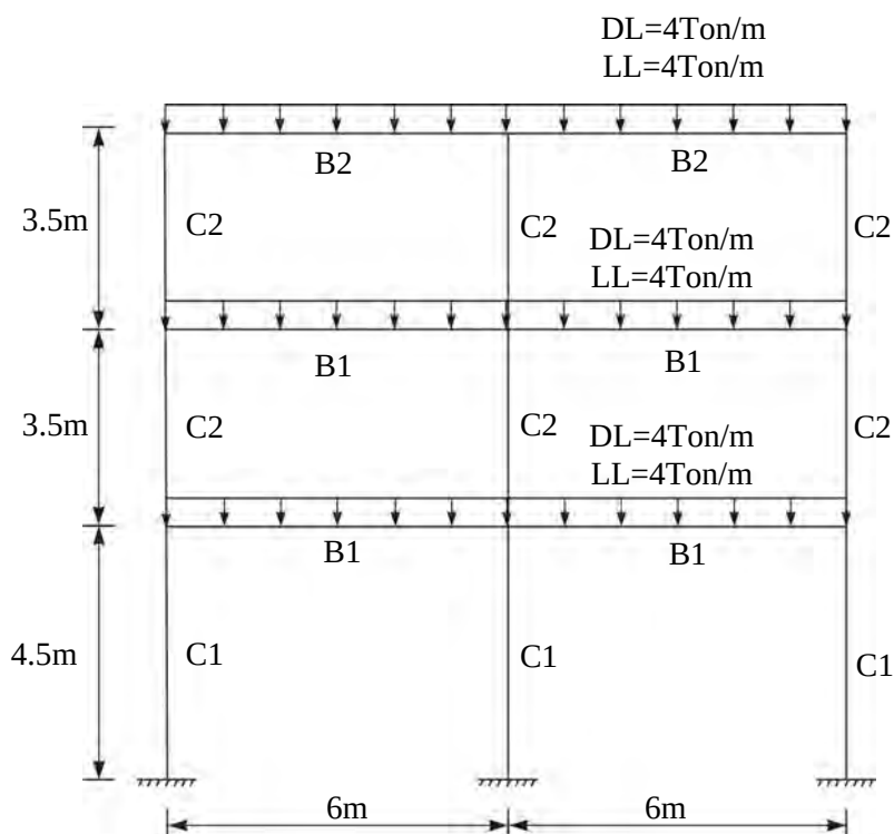
شکل ۳۰-۶ پیکربندی و بارگذاری ثقلی قاب خمشی بتنی
