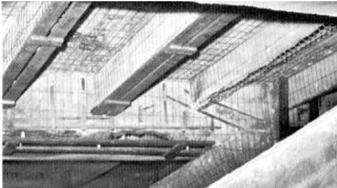
شکل ۳-۳-۲- افزایش ضخامت دال از قسمت تحتانی با شاتکریت
