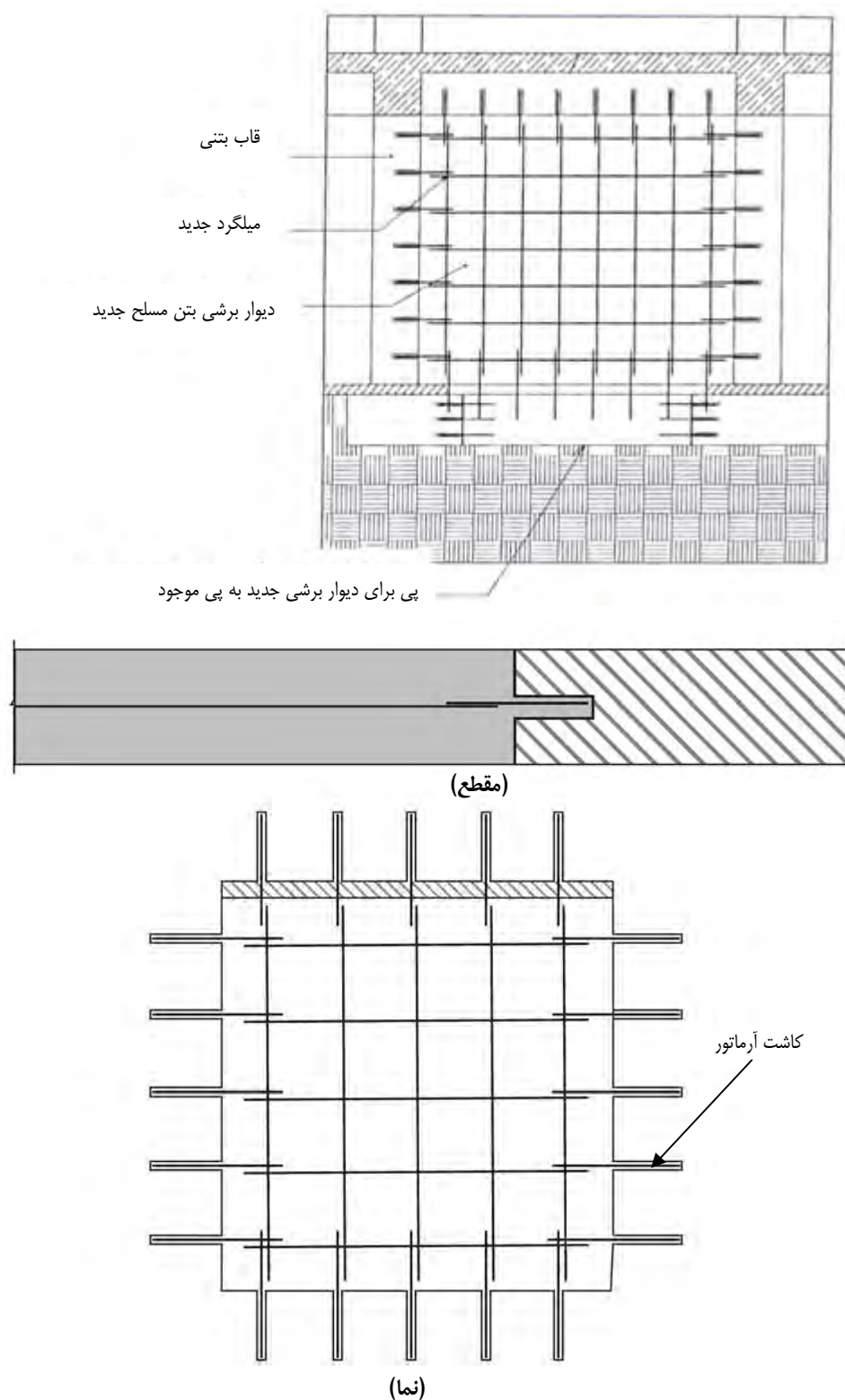
شکل ۴-۴۸- اضافه کردن دیوار برشی جدید در یک قالب بتنی
