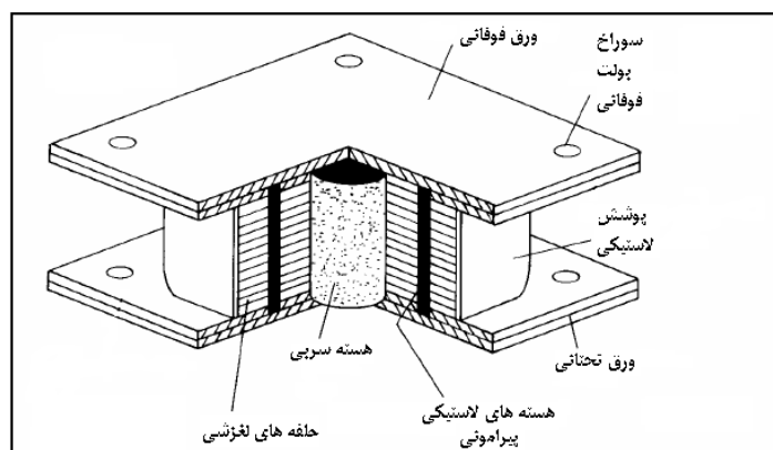
شکل ۶-۱۰ - جداگر R-FBI
