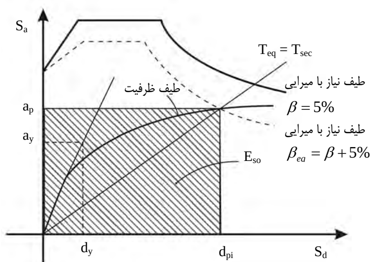
شکل ۵-۱- مشخص کردن نقطه عملکرد و جابجایی هدف
