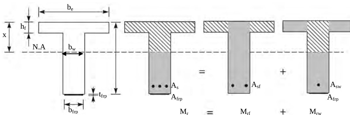
شکل ۱۲-۴-۲ نحوه تفکیک لنگر مقاوم تیر T شکل
