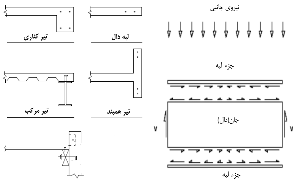
شکل (۸-۱) نمایش انواع اجزای لبه
