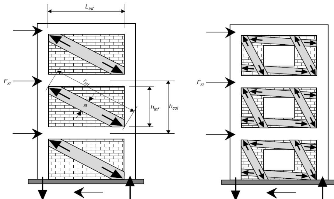
شکل (۵-۸): جایگزینی میانقاب با دستک فشاری معادل
