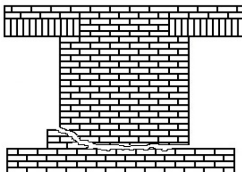
شکل (۷-۳): مود خرابی لغزش سطوح اتصال
