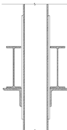
شکل (۵-۱۵): اتصالات خورجینی سستی با نبشی پایین
