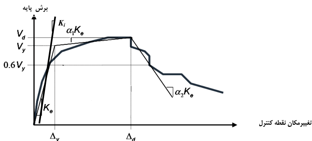
شکل (۵-۳): منحنی ساده شده تغییرمکان سازه
